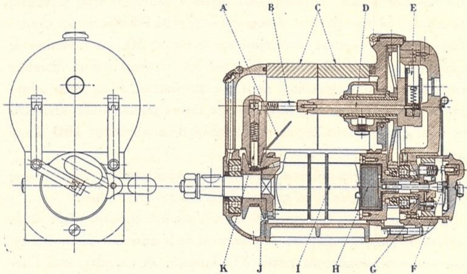
Fig. 11. — Magnéto.
